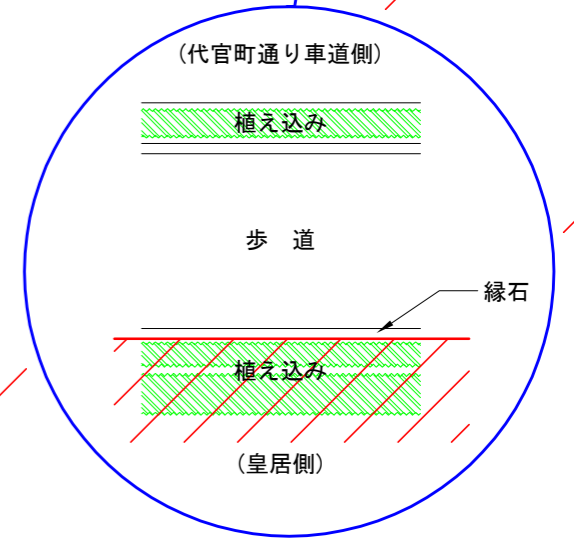
代官町通り沿い詳細図
